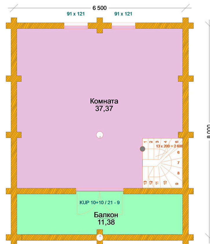
План 2-го этажа
